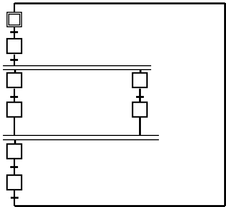
Langage PB / grafcet esclave
