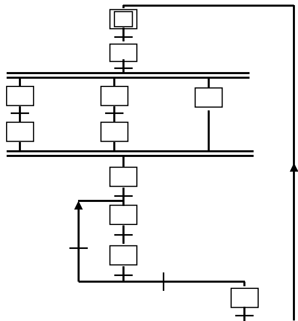
Langage PB / grafcet esclave / diapo 25
