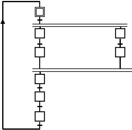
Analyse / grafcet maître niveau 1 / diapo 10
