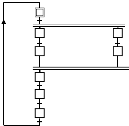
Langage PB / grafcet maître
