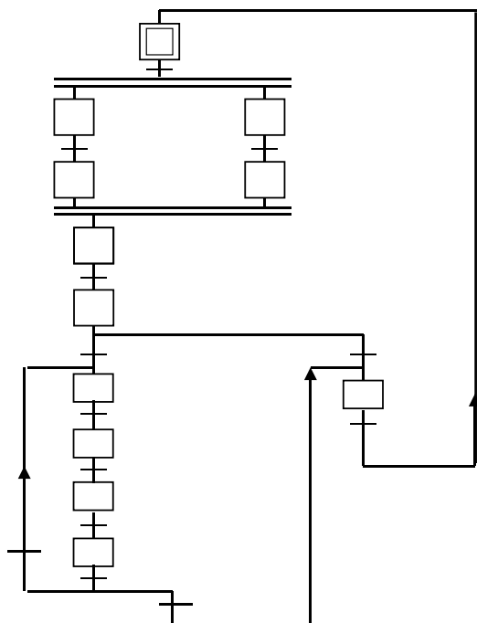
Langage PB / grafcet maître / diapo 23 et 24
