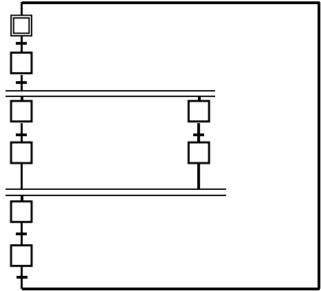
Analyse / grafcet esclave niveau 1 / diapo 11
