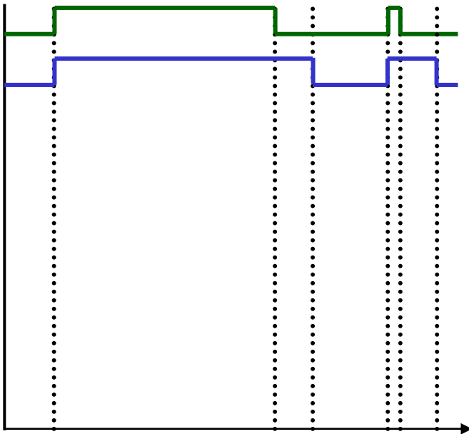
Temporisation à l'enclenchement et au déclenchement
